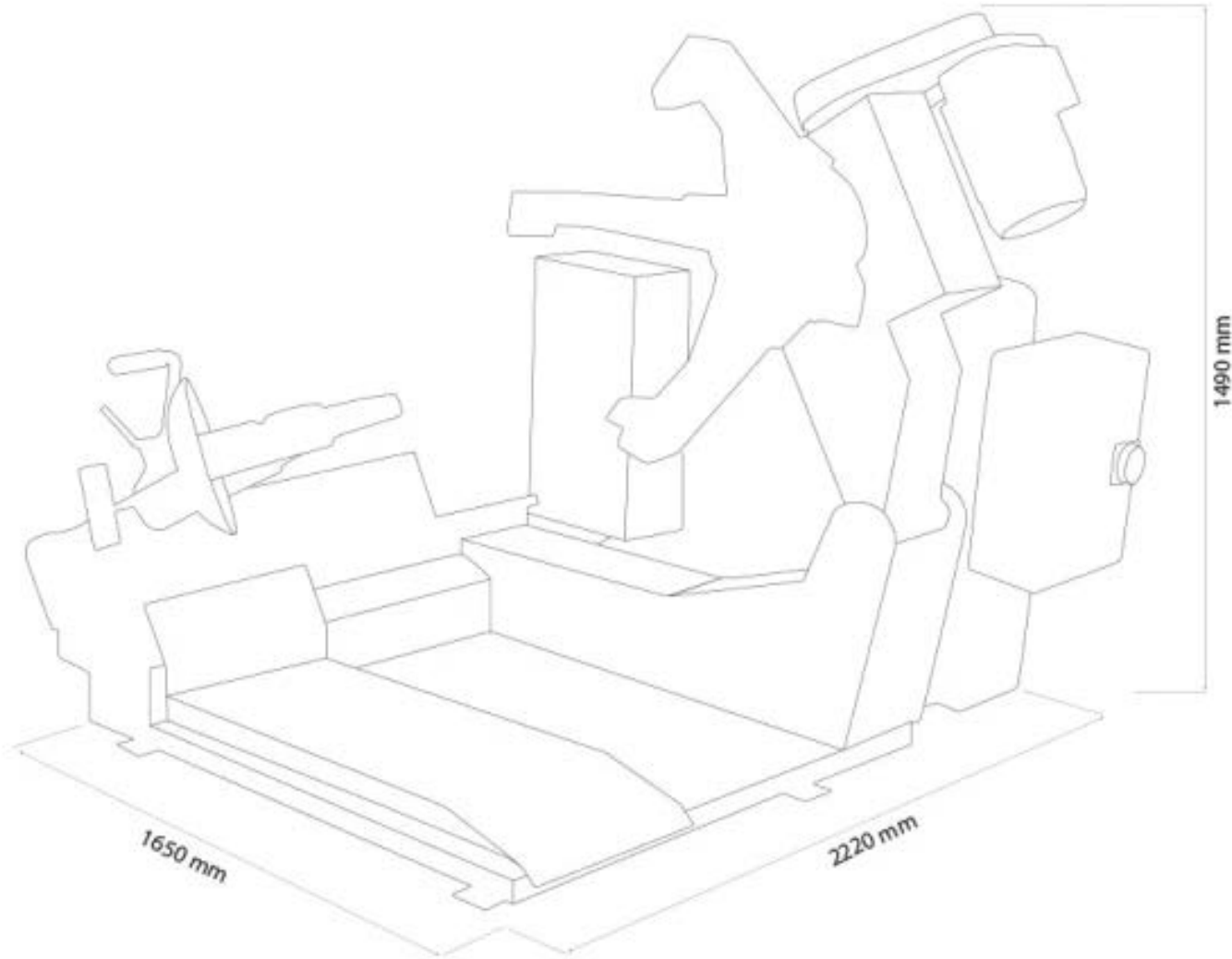
Reifenmontiermaschine LKW 151
